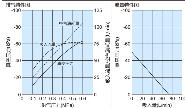
ZH15 □ L
