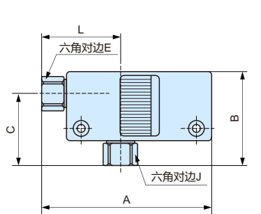
<内螺纹型>
