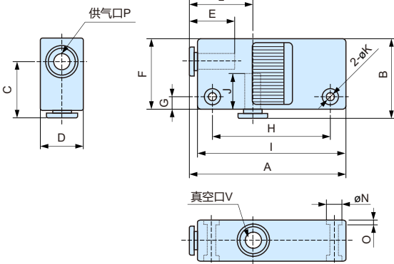
<快速接头型>
