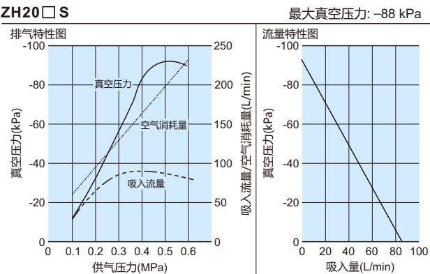
<快速接头型>
